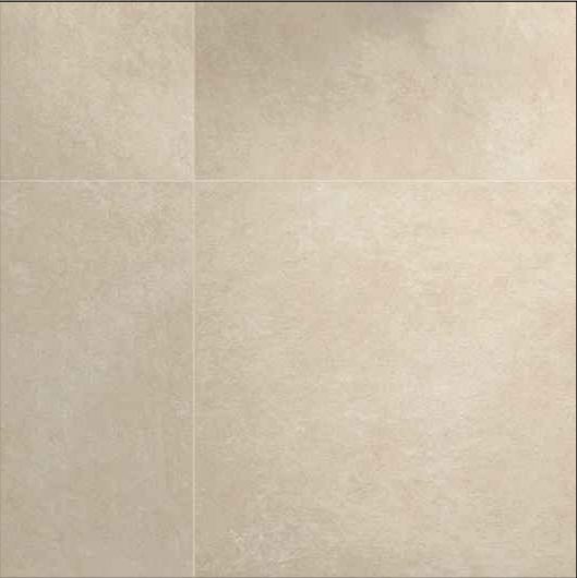
P3 - KERAMICKÝ OBKLAD - REF. VÝR. ASSO UNI 25 BEIGE - ROZMĚR: 60x60cm, TL. 1cm - BARVA: SVĚTLE BÉŽOVÁ - EPOXIDOVÁ SPÁROVACÍ HMOTA V ODSTÍNU OBKLADU (SVĚTLE BÉŽOVÁ) - REKTIFIKOVANÁ HRANA
